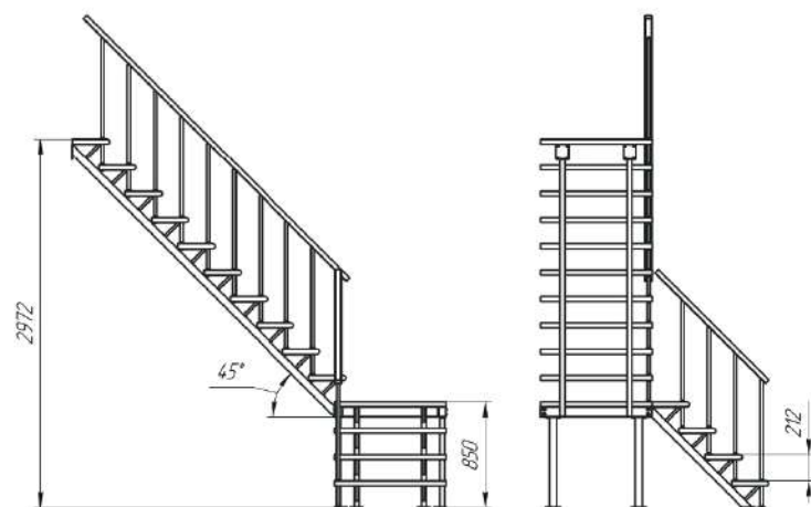
Рисунок 1. Лестница внутриквартирная ЛЕС-05-3.
