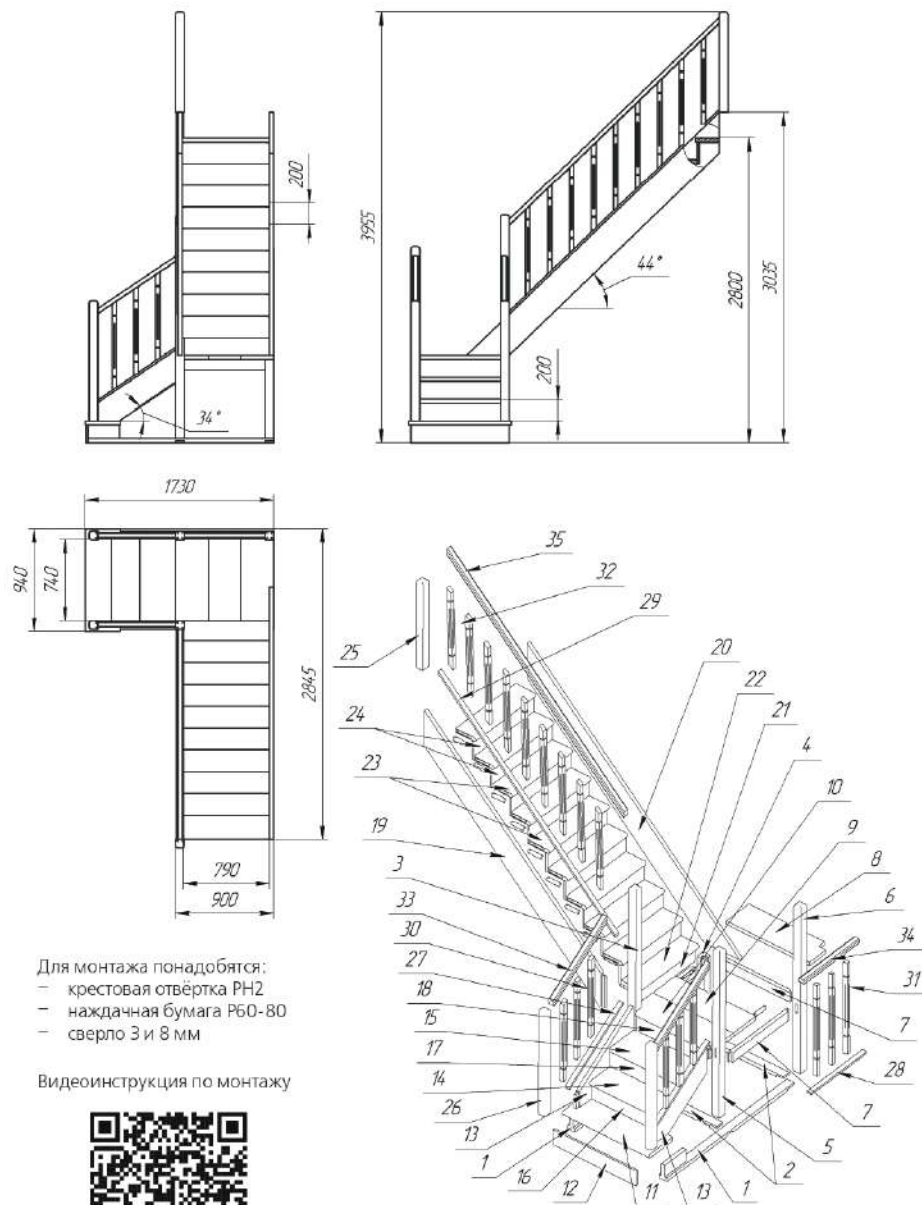
Рисунок 1. Лестница внутриквартирная ЛЕС-04.
